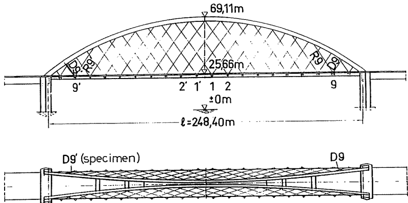
Fig. 2. Fehmarnsundbridge-survey
