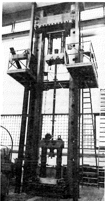
Fig. 1. Test setup
