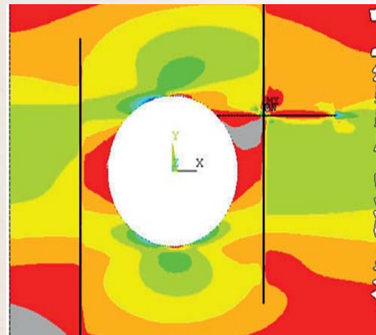
Experimentelle Untersuchungen und Finite-Elemente-Simulationen zum Rissfortschritt und zur Bewehrung von Holzbauteilen
